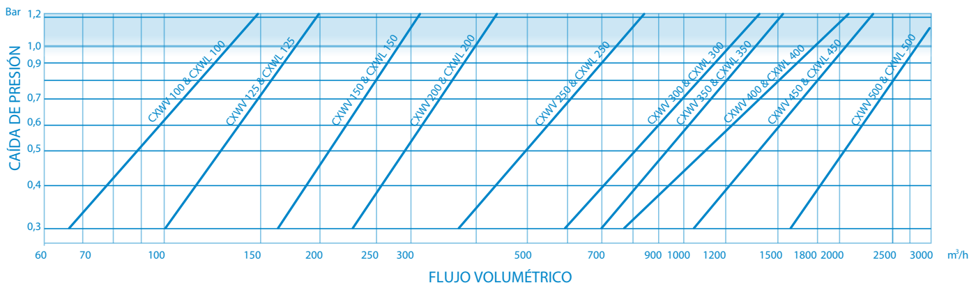
GRÁFICO DN100-500
